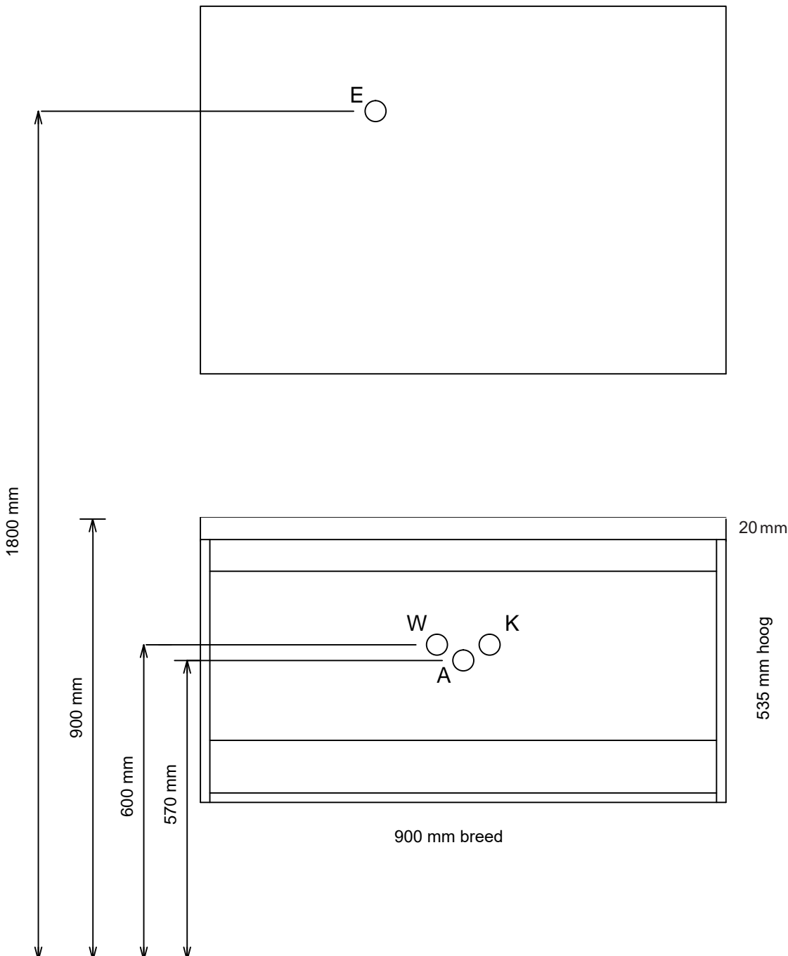
Vooraanzicht
